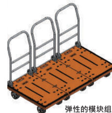
弹性的模块组合(只适用DS-5) Module combination(For DS-5 only)
