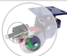
AK刹 Swivel W/Center Lock(AK type) & 轮子可附塑料防尘盖(供选择) Plastic Thread Guard(optional)
